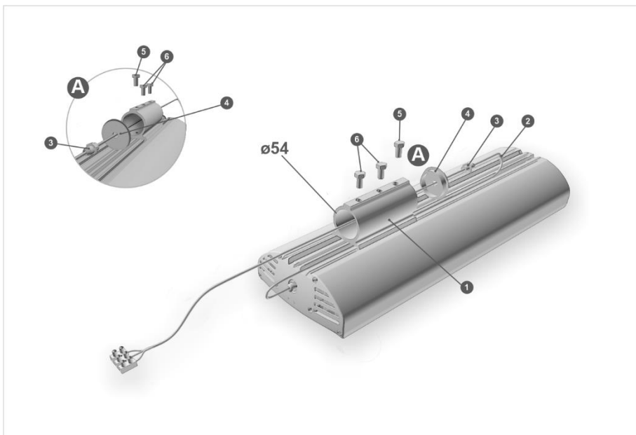
Рисунок 1. Схема монтажа светильника GSFO.
