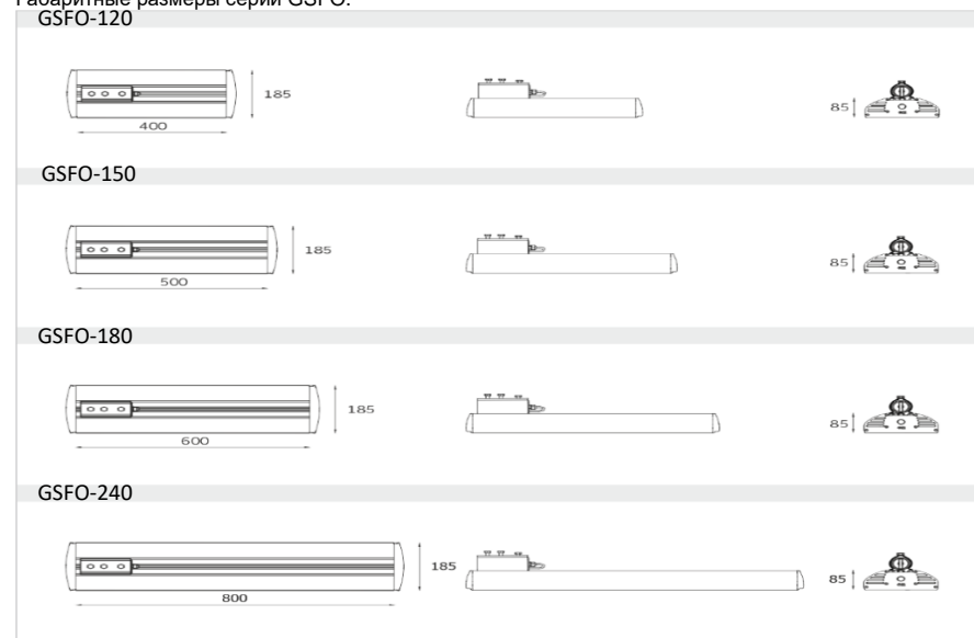
Габаритные размеры серии GSFO.
